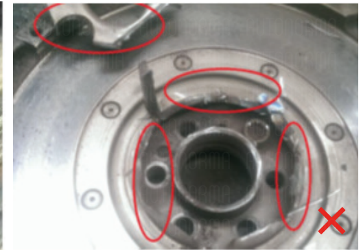
Beschädigtes Getriebe
